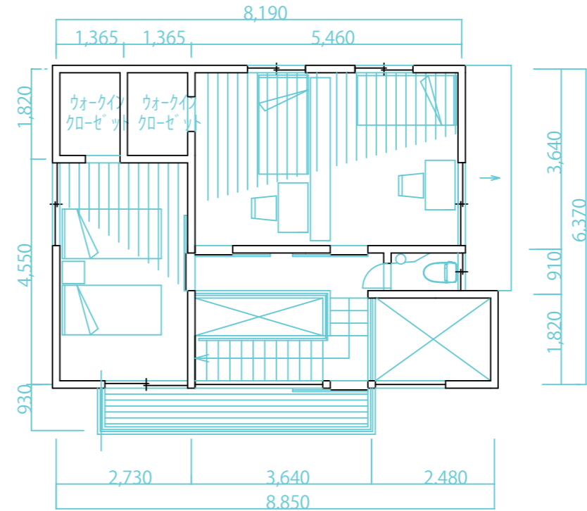
2階平面図
