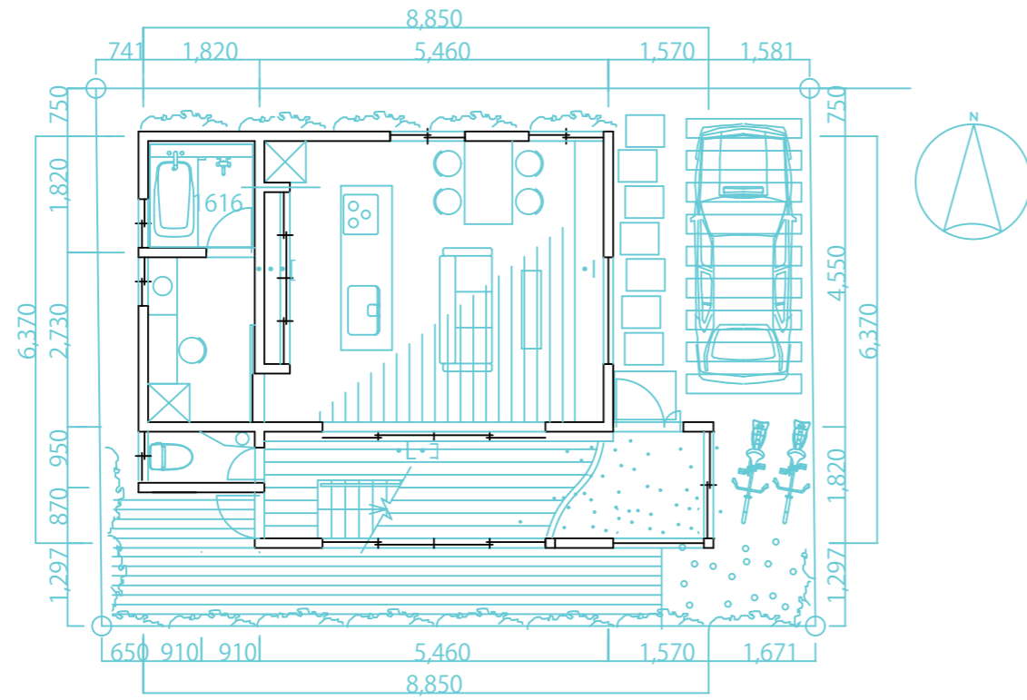
1階平面図
