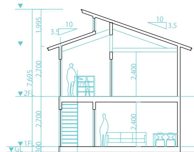
断面図
